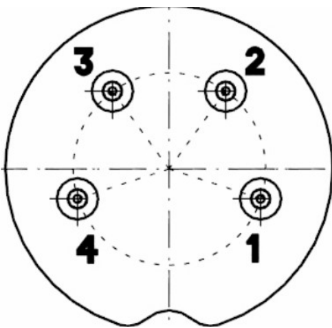
Cable side
